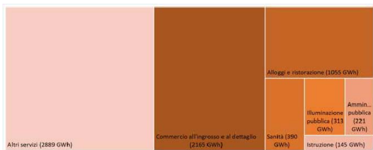
Figura 3.61 - Consumi finali di energia elettrica nel settore terziario in Veneto nel 2020, dettaglio per comparto. Fonte: elaborazione RSE su dati statistici TERNA [8].
