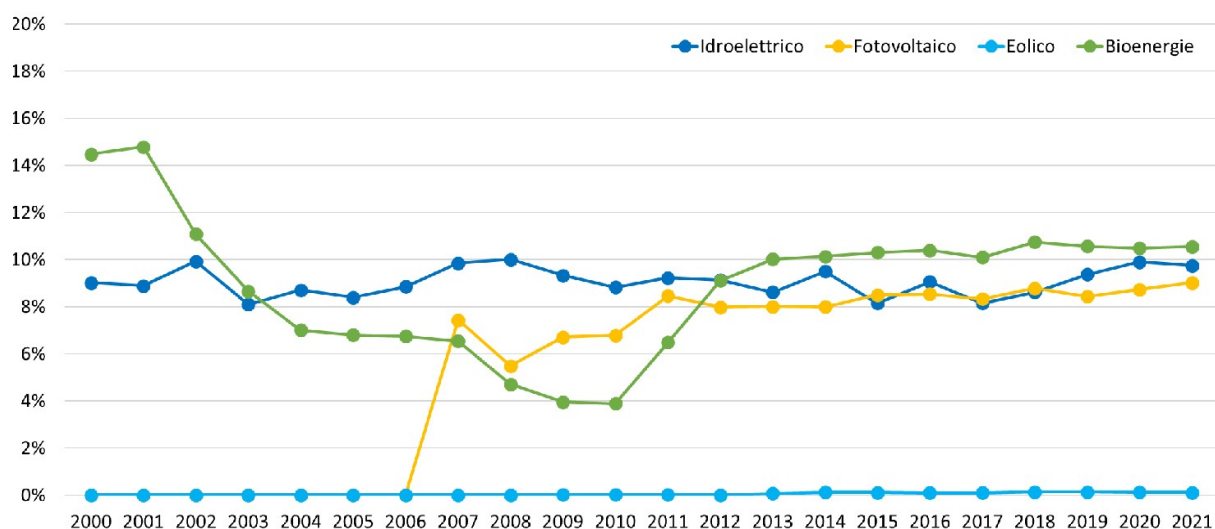
Figura 9: Serie storica della percentuale di produzione lorda di energia elettrica da FER, per fonte, in Veneto rispetto alla produzione totale nazionale per fonte. Fonte: elaborazione RSE su dati statistici TERNA
