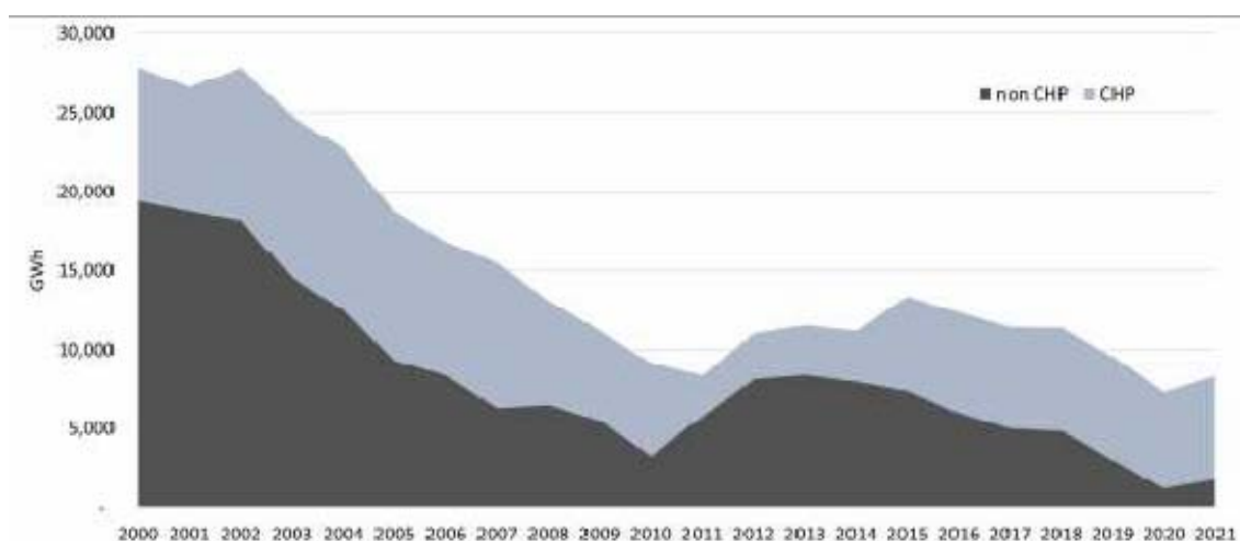
Figura 3.39 - Serie storica della produzione lorda di energia elettrica da impianti termoelettrici in Veneto, dettaglio cogenerazione. Fonte: elaborazione RSE su dati statistici Terna [8].
