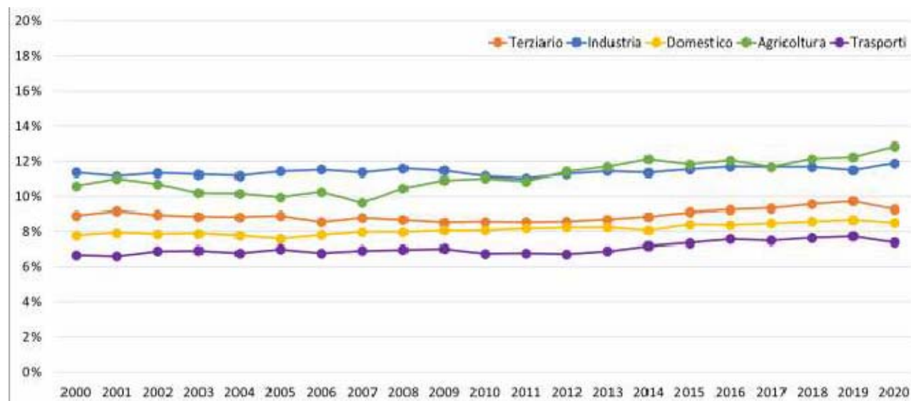
Figura 3.58 - Serie storica della percentuale dei consumi di energia elettrica, per settore, in Veneto rispetto ai consumi totali nazionali per settore. Fonte: elaborazione RSE su dati statistici TERNA [8].
