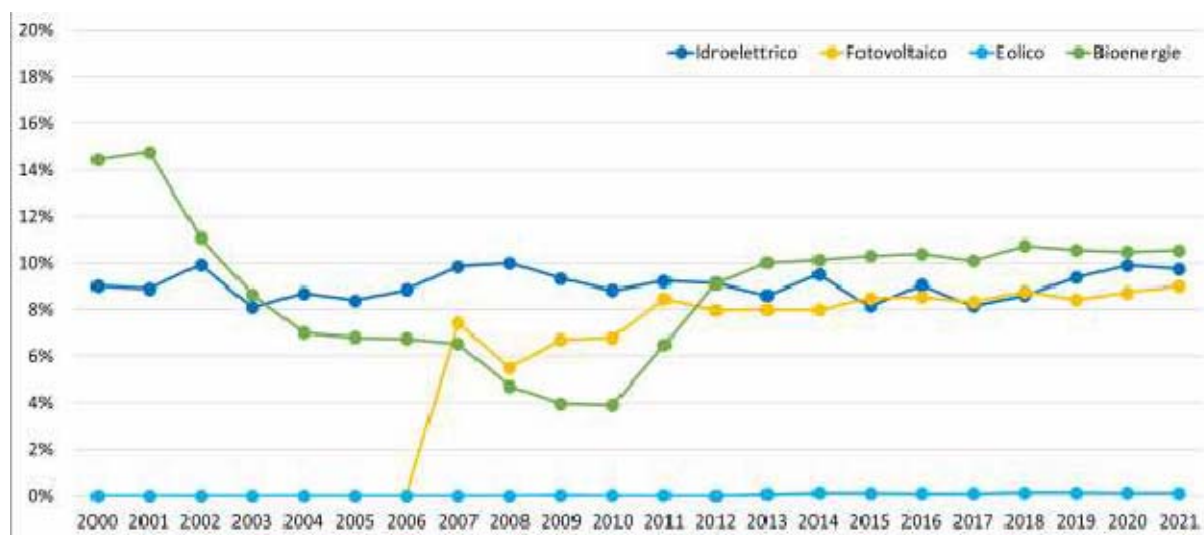
Figura 3.44 - Serie storica della percentuale di produzione lorda di energia elettrica da FER, per fonte, in Veneto rispetto alla produzione totale nazionale per fonte. Fonte: elaborazione RSE su dati statistici TERNA [8].
