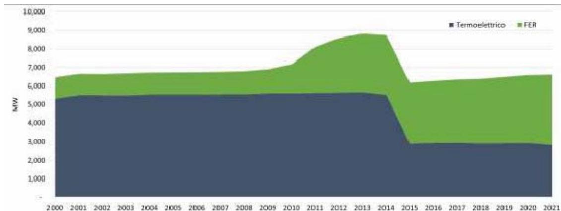
Figura 3.34 - Serie storica della capacità lorda di generazione elettrica in Veneto. Fonte: elaborazione RSE su dati statistici TERN [8].
