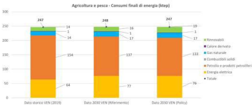
Figura 4.24 – Consumi finali del settore agricolo per fonte: confronto tra il dato storico 2019 e i risultati al 2030 degli scenari.
