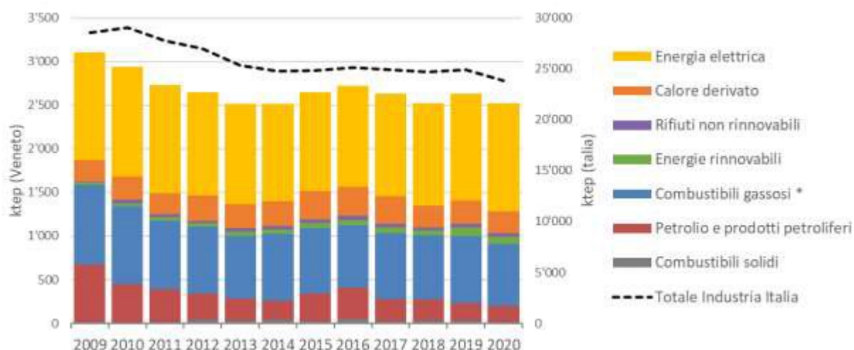
Figura 3.65 – Consumi finali del settore industriale in Veneto (per fonte) e in Italia (totali). * Gas naturale e gas manufatti. Fonte: elaborazione RSE su dati ENEA e Eurostat.
