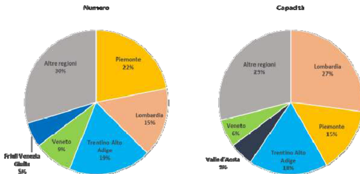
Figura 3.50 - Distribuzione percentuale della numerosità e della potenza installata degli impianti idroelettrici, anno 2021. Fonte: elaborazione RSE su dati TERN [8] e GSE [9].
